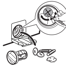
7. Verwijder indien noodzakelijk pluizen en andere voorwerpen uit de filterholte. Verzeker u ervan dat de pompwaaier onbelemmerd kan ronddraaien. Als hij niet roteert: neem contact op met een erkend servicecentrum.
